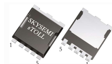
sTOLL
